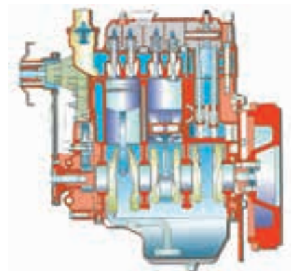
Velkokapacitní dieselové traktory podávají optimální výkon již při nízkých otáčkách. Tím je dosaženo konstantně vysokého maximálního točivého momentu – tedy výkonu a odpovídající rezervy tam, kde je zapotřebí.
